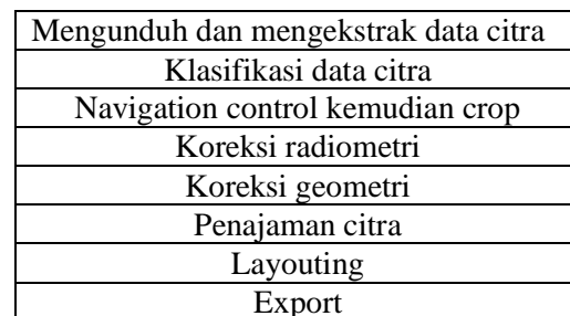
Gambar 2. Diagram Alir Pengolahan Data NOAA/AVHRR
